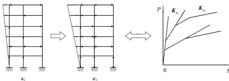
图3.2 非线性构形状态转移过程示意图
